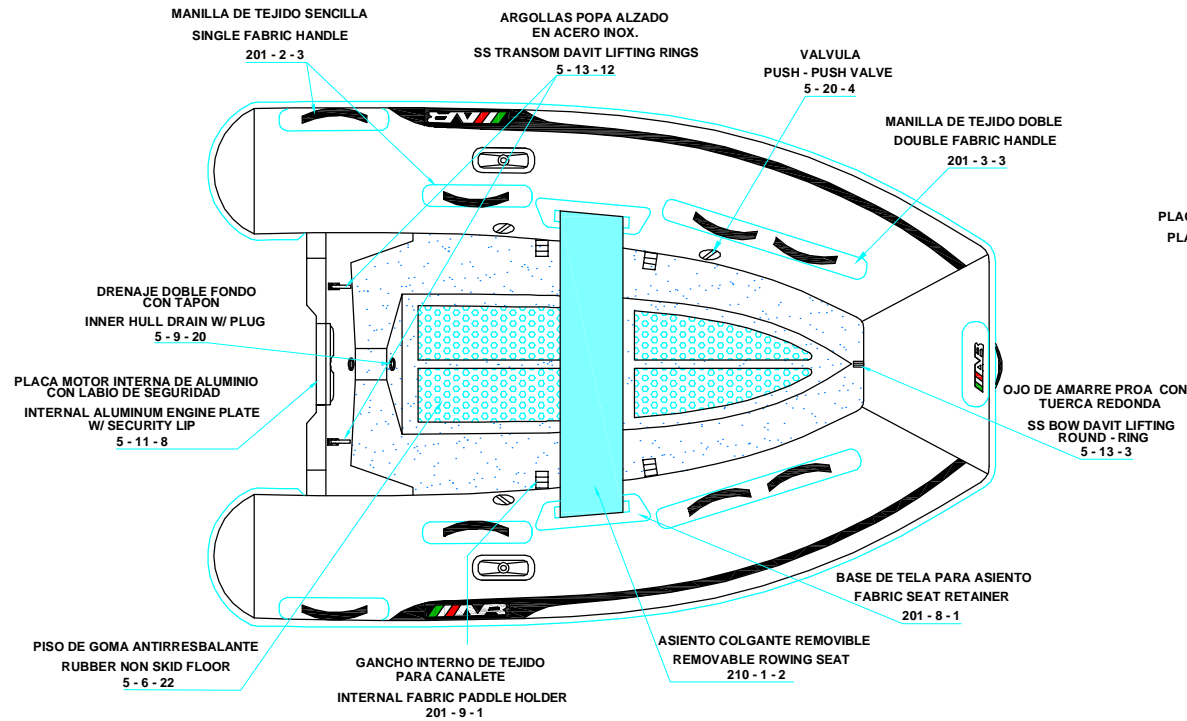
PLANT VIEW VISTA EN PLANTA
