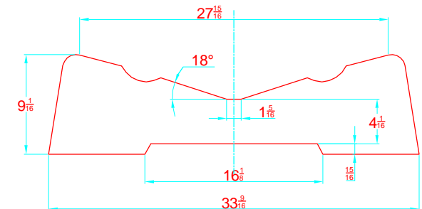
TRANSVERSAL SECTION "B" SECCION TRANSVERSAL "B"
