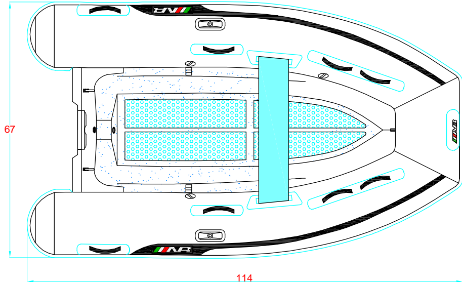
PLANT VIEW VISTA EN PLANTA
