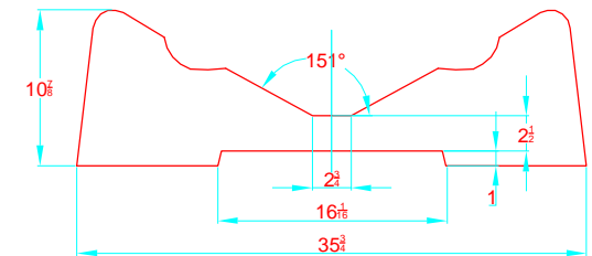
TRANSVERSAL SECTION "B" SECCION TRANSVERSAL "B"
