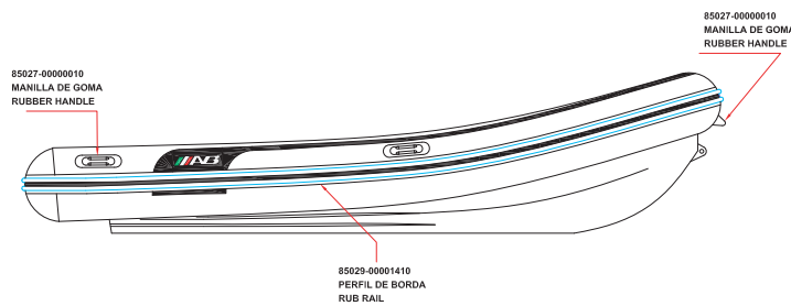
LONGITUDINAL PROFILE
