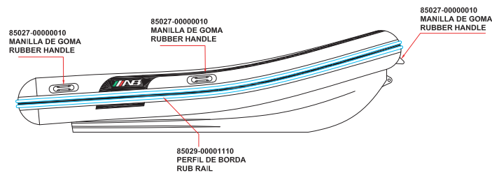
LONGITUDINAL PROFILE
