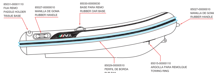
LONGITUDINAL PROFILE
