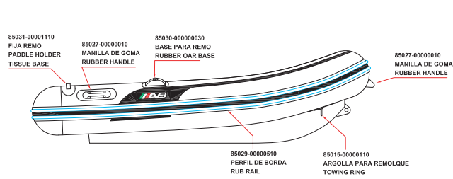
LONGITUDINAL PROFILE
