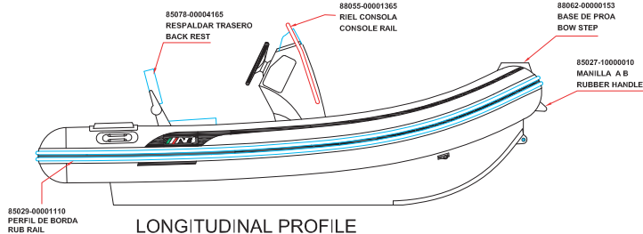
LONGITUDINAL PROFILE
