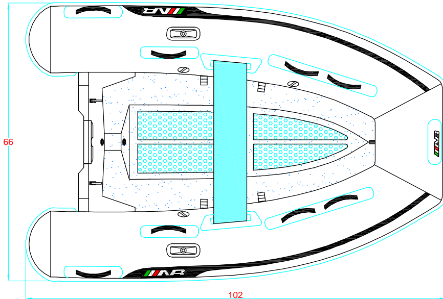
PLANT VIEW VISTA EN PLANTA
